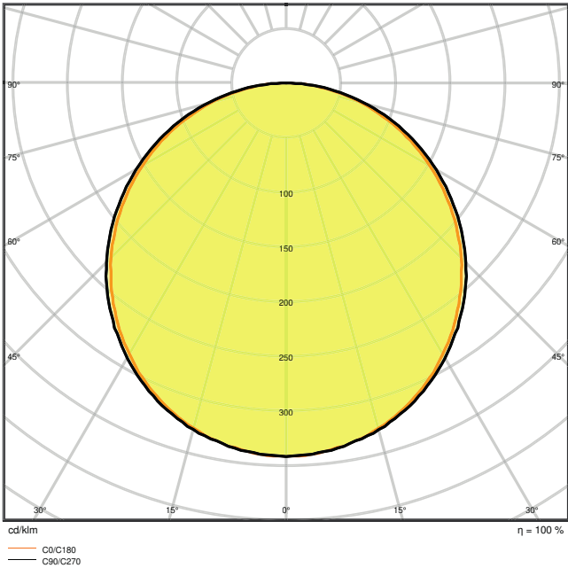
PL PFM DALI 600 40W 4000K
